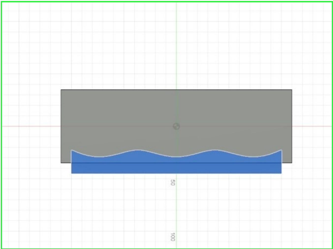
"Sketch 3 plano anterior > Create > Project tapa superior"
