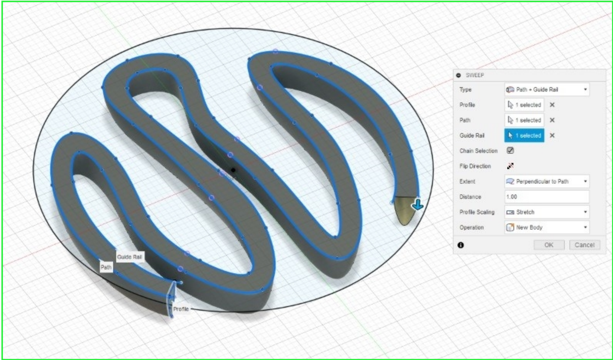
"Sweep splines con Guide Rail y Stretch profile"
