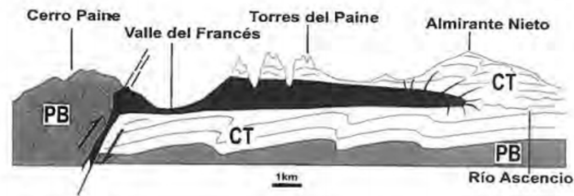
FIG. 3. Diagrama que muestra una sección esquemática del Granito de las Torres del Paine, desde el Cerro Paine (oeste) hasta el río Ascencio (este). Ubicación aproximada es la de la sección A-A en la figura 2. PB- Formación Punta Barrosa; CT- Formación Cerro Toro.
